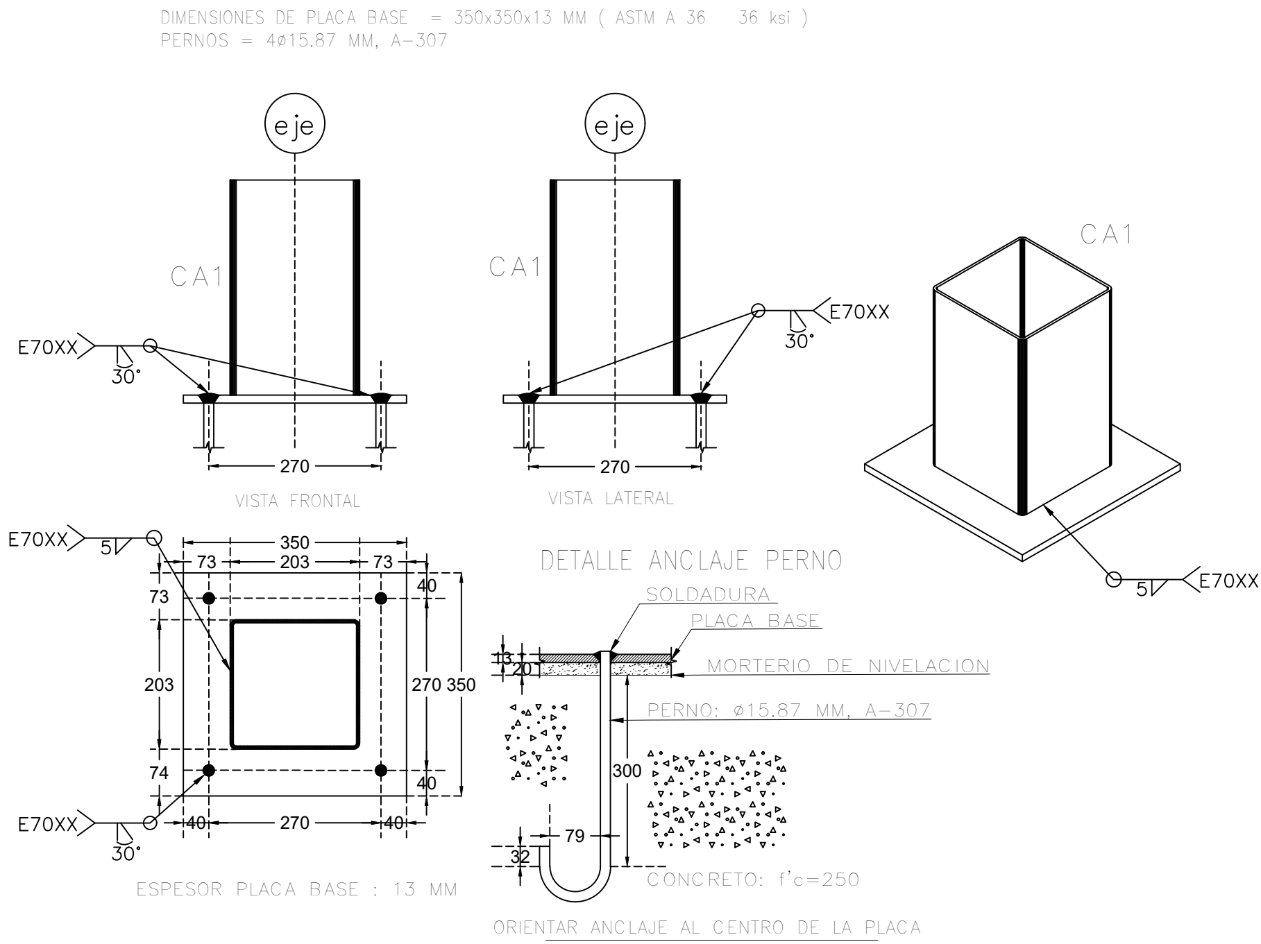
DETALLE PLACA BASE PLB -1
