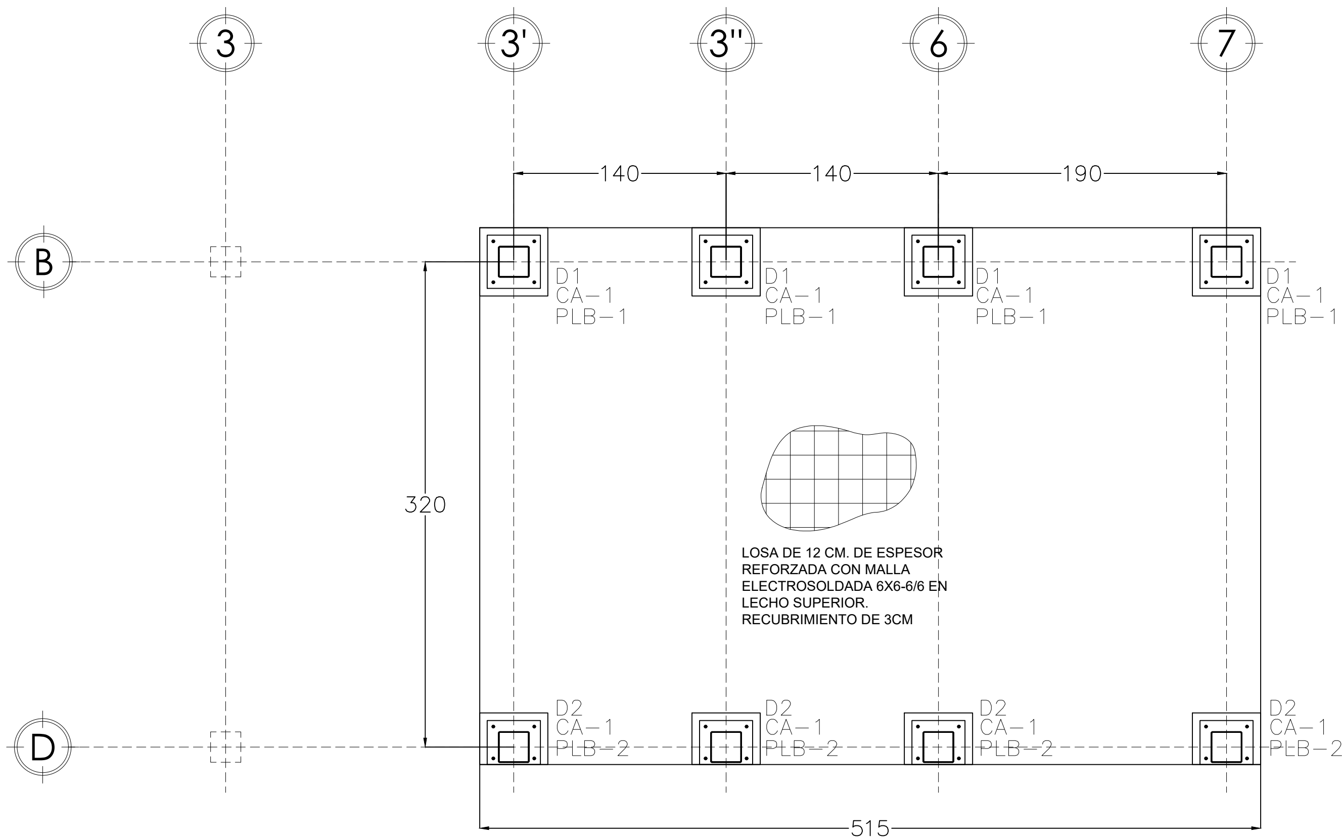
LOSA DE CIMENTACIÓN 1
