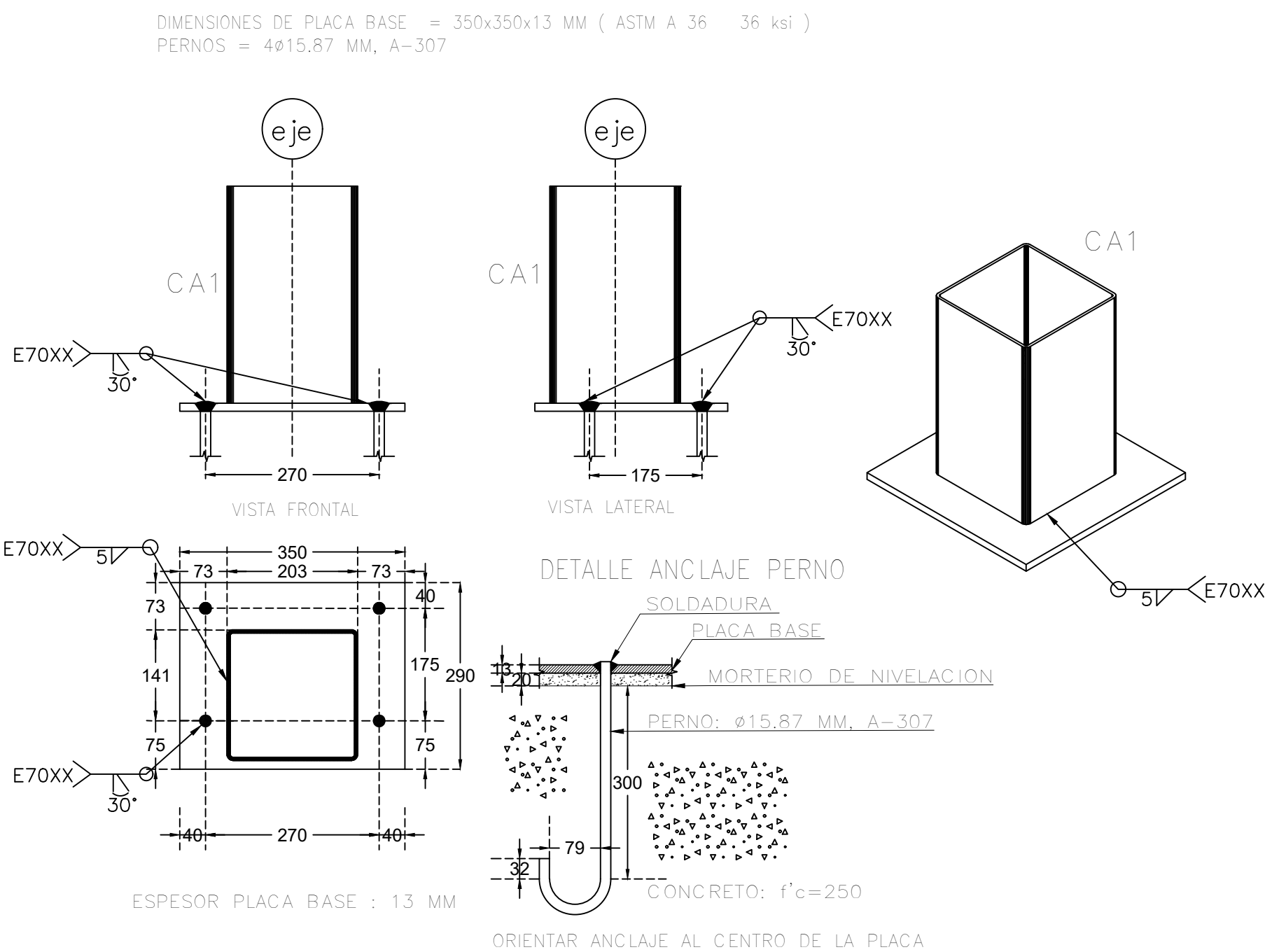
DETALLE PLACA BASE PLB -2
