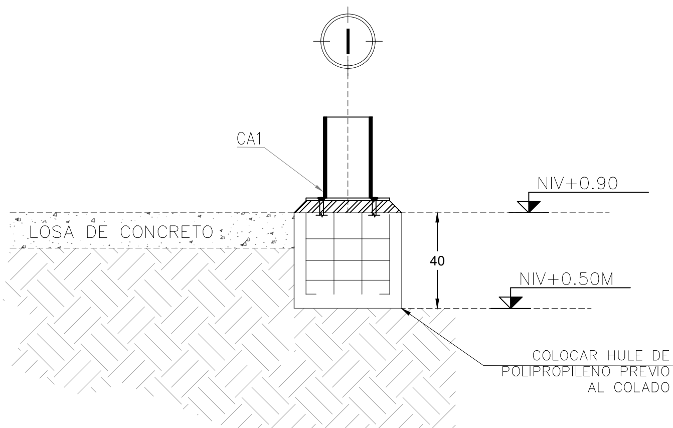
DETALLE - CONEXIÓN COLUMNA ALZADO
